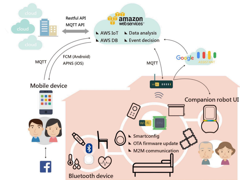
圖 1. 「天才家居」發展完成之整體資訊架構
